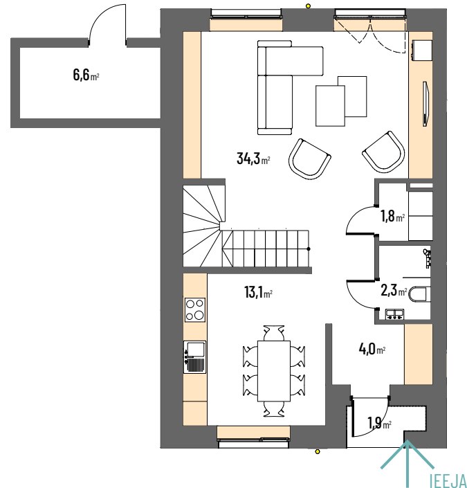
1. stāva plāns
