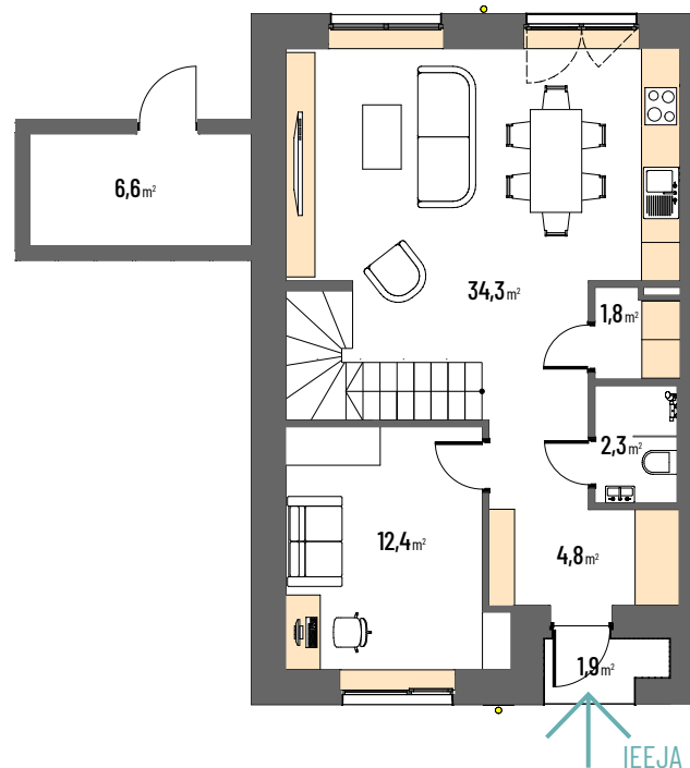
1. stāva plāns
