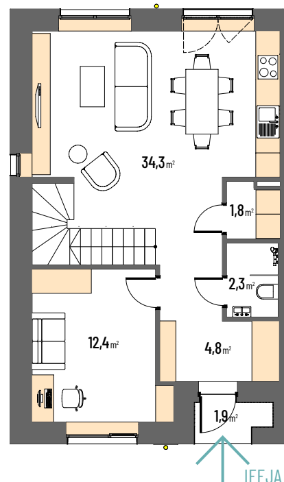
1. stāva plāns
